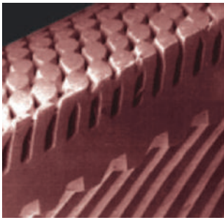
Структура медных трубок затопленного испарителя
