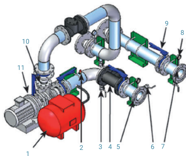
Гидравлический модуль
