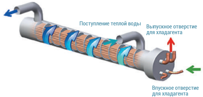
Кожухотрубный теплообменник
