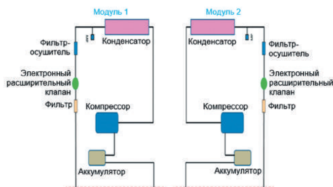
Двухконтурный компрессорно-конденсаторный блок, состоящий из двух модулей
