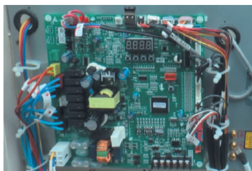
Плата управления
