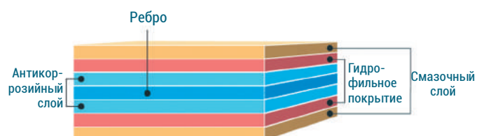
Двустороннее антикоррозийное покрытие алюминиевых ребер конденсатора
