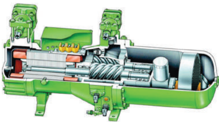
Двухвинтовой компрессор
