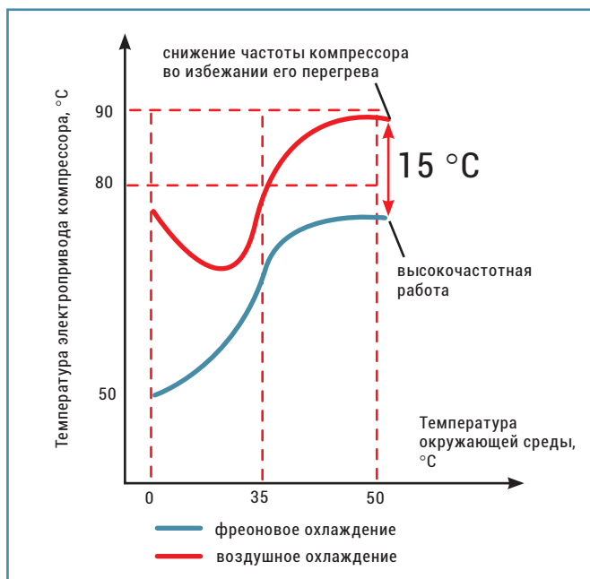
Температура электропривода при использовании фреонного и воздушного охлаждения
