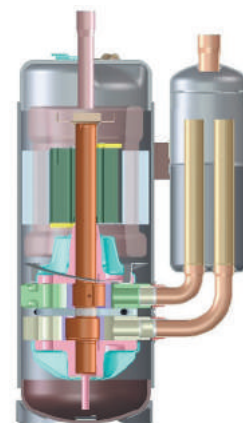
Двухроторный компрессор
