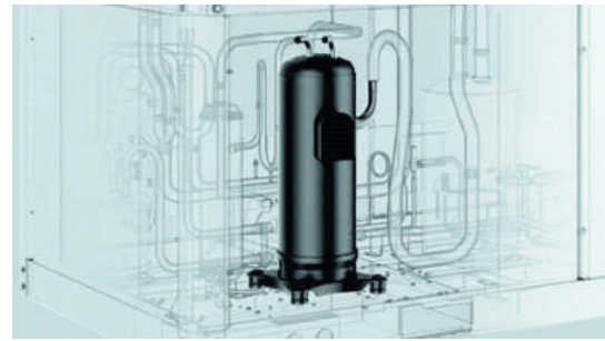
Герметичный спиральный компрессор
