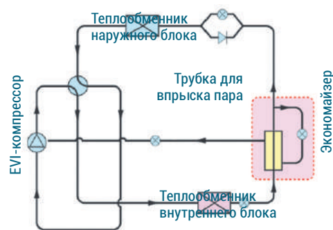
Схема теплового насоса (чиллера) с технологией EVI
