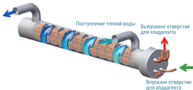
Кожухотрубный испаритель
