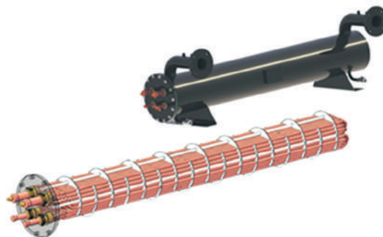
Кожухотрубный испаритель
