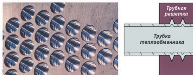
Трубная решетка
