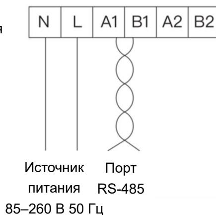
Схема подключения
