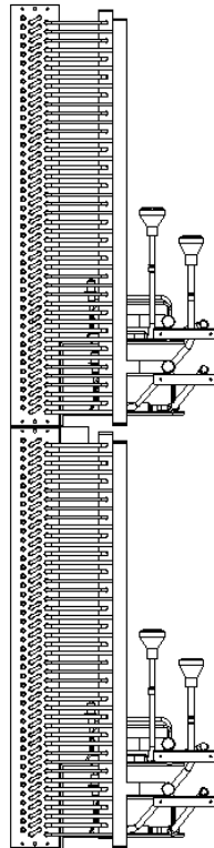
Испаритель воздухообрабатывающих установок производительностью 250—270/286—310 кВт (110/125 л. с.) (с дросселирующим устройством)
