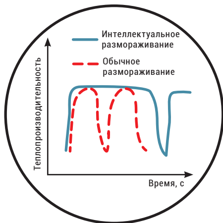
Теплопроизводительность chillера при стандартном и умном размораживании
