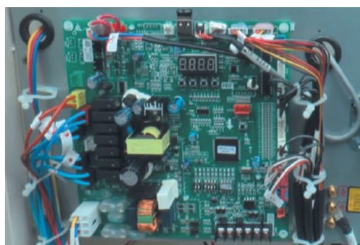
Плата управления
