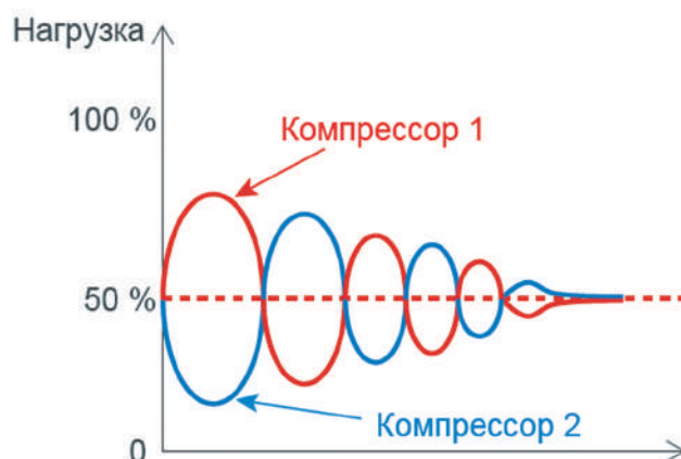
Выравнивание нагрузки между компрессорами
