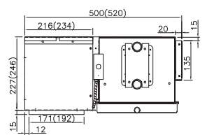
Пленум-бокс установлен снизу (размеры TCR1200J указаны в скобках)
