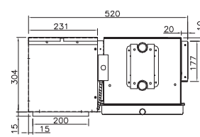
Пленум-бокс установлен снизу
